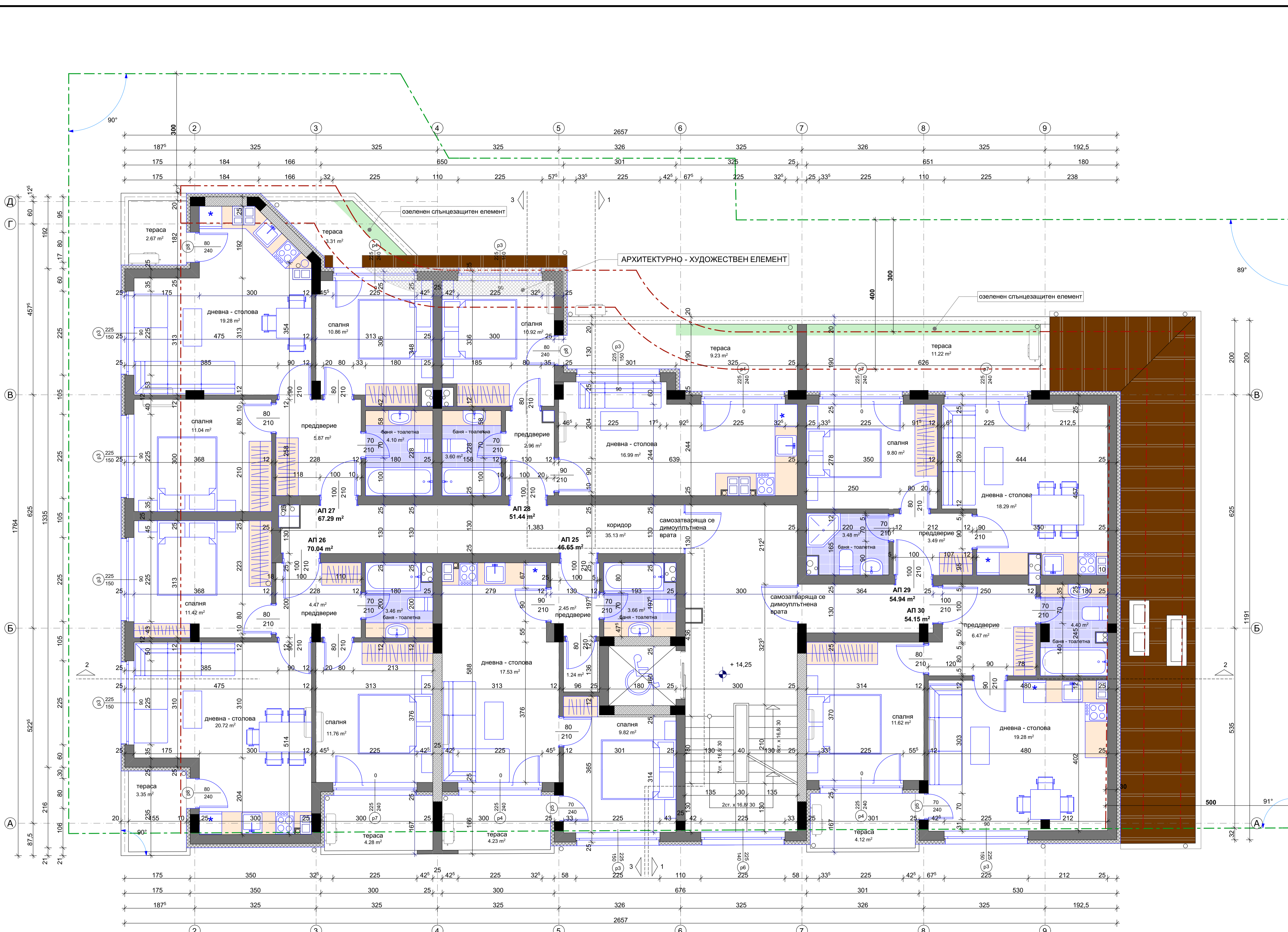
РАЗПРЕДЕЛЕНИЕ ПЕТИ И ТАВАНСКИ ЕТАЖ М 1:50
